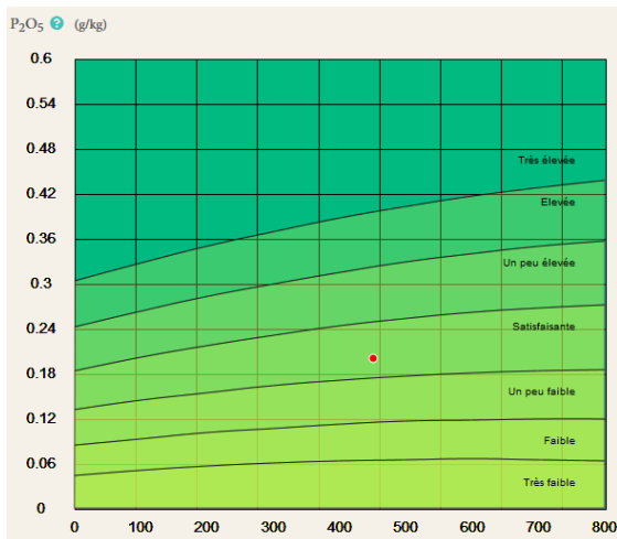
Figure 2 : Fertilité en P_2O_5 (source : Inra LAS)
